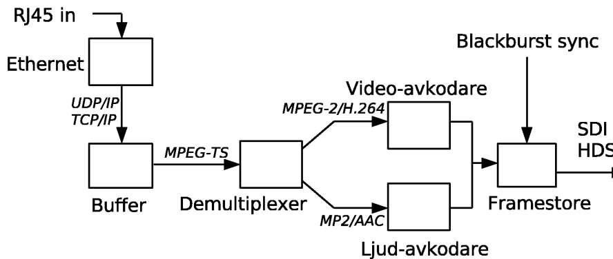
Figur 2.1: teknisk översikt
