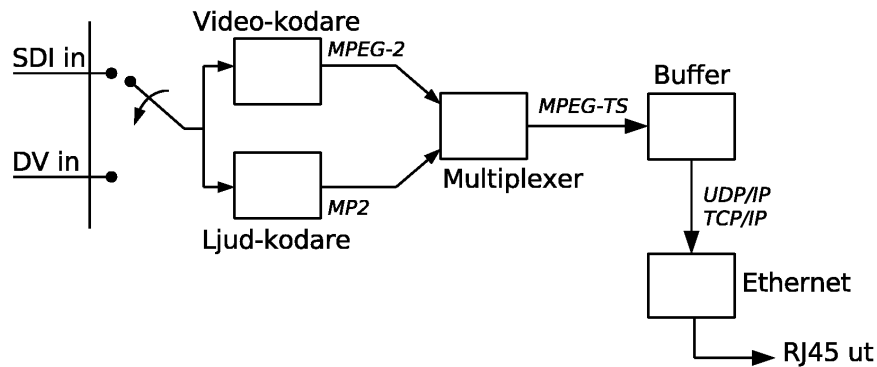
Figur 3.1: teknisk översikt
