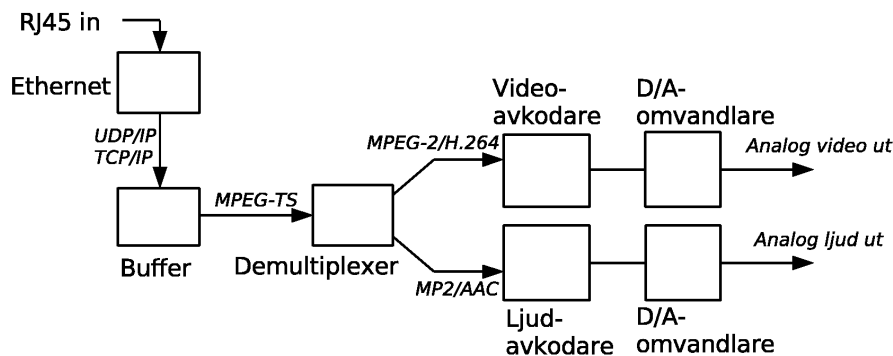
Figur 2.1: teknisk översikt
